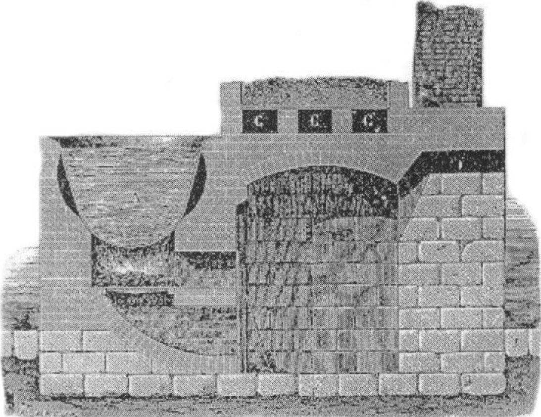
Chaudière pour l'extraction du salpêtre
